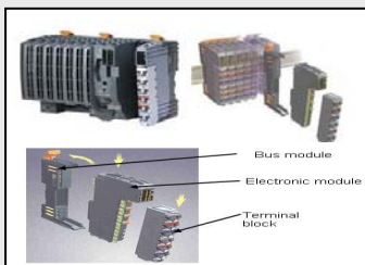
Figure 2 : ALSPA MFC3000 - Contrôleur multifonction basé sur le standard industriel
